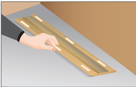
1. Adhiere la cinta bifaz en el dorso del junquillo con cortes de 2 cm/ 1" cada 40 cm/ 16" y a no menos de 20 cm/ 8" de los extremos del perfil.
